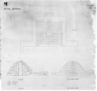
[19] Section by Stanislas Jasinski Le Corbusier, Musée Mondial (1929), FLC, doc nr. 24510
